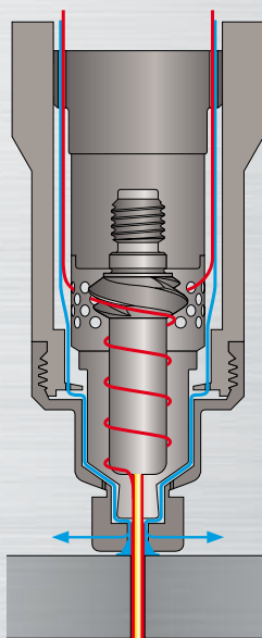
LC105 toortsonwerp met sleepmondstuk
